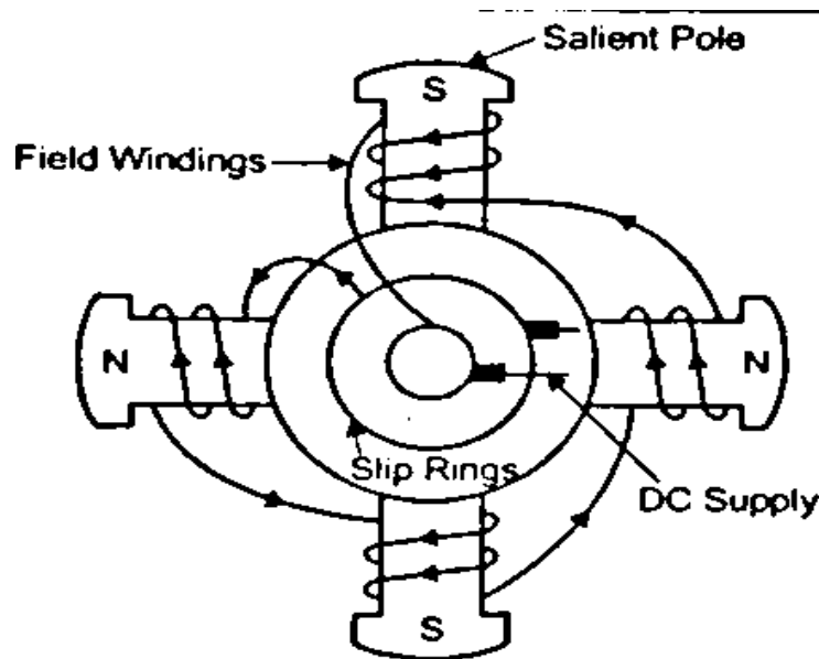
Fig 4.33 Salient pole rotor
